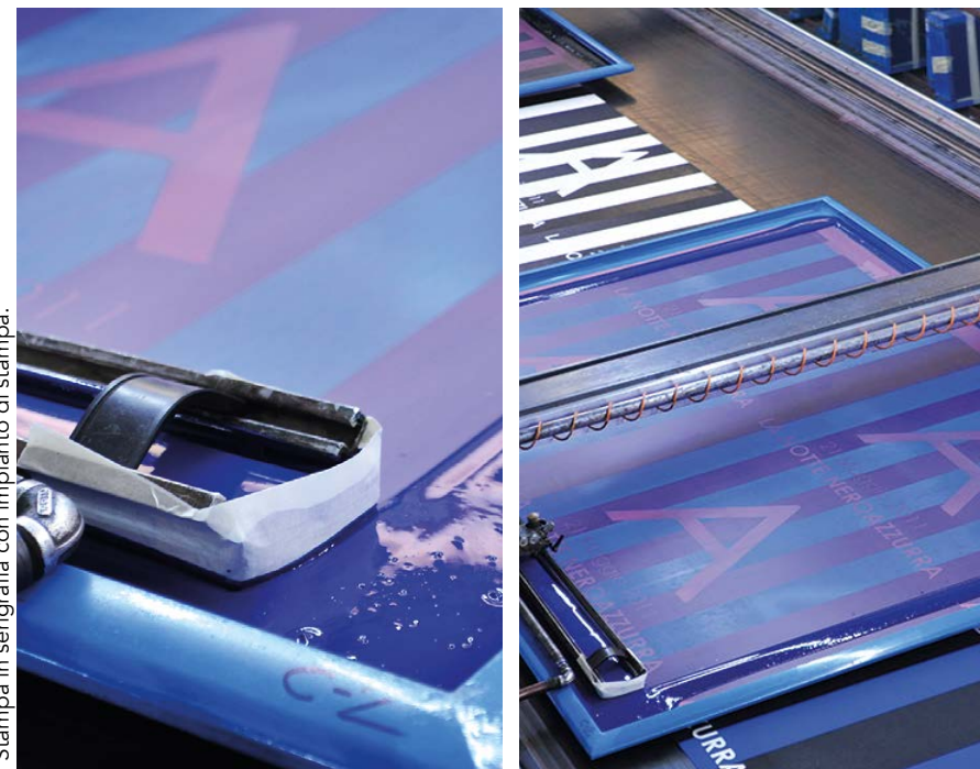
Stampa in serigrafia con impianto di stampa.
